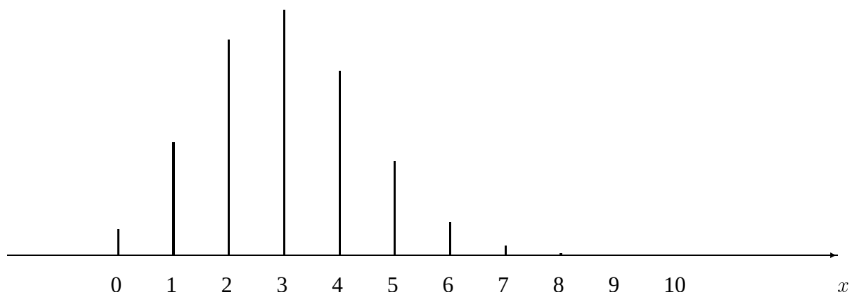
Figura 3.2: Funzione di probabilità distribuzione binomiale di parametri n = 10 e p = 0.3 .
