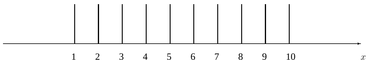
Figura 3.1: Funzione di probabilità di distribuzione uniforme discreta su \{1, 2, \dots, 10\} .
