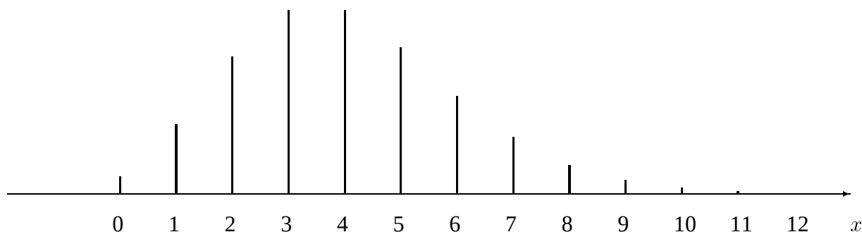
Figura 3.3: Funzione di probabilità distribuzione di Poisson con parametro \lambda = 4 .
